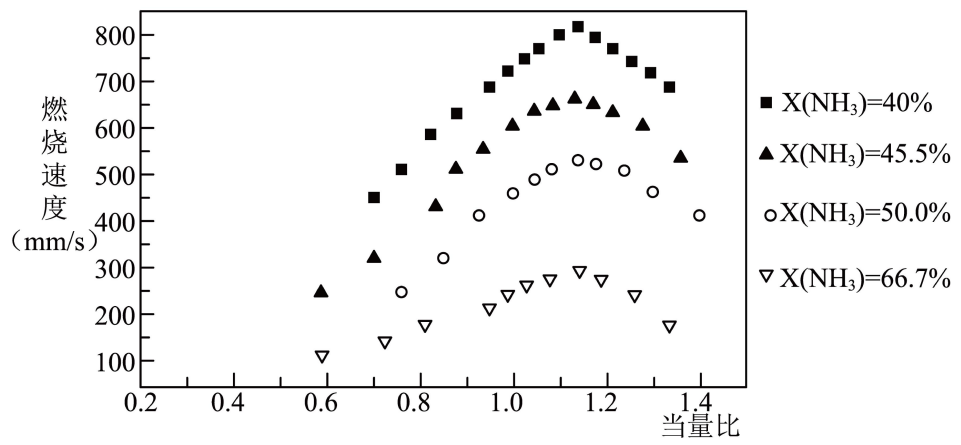
图3 不同当量比下氨气/氢气/空气的燃烧速度
